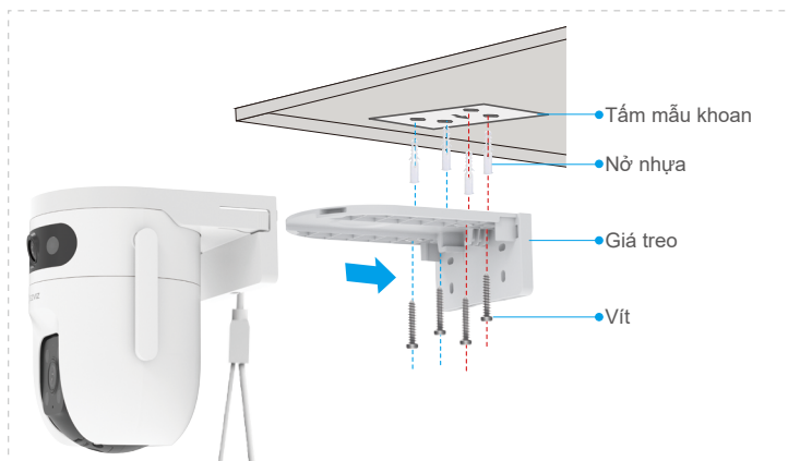
Hình 1 Gắn trần
