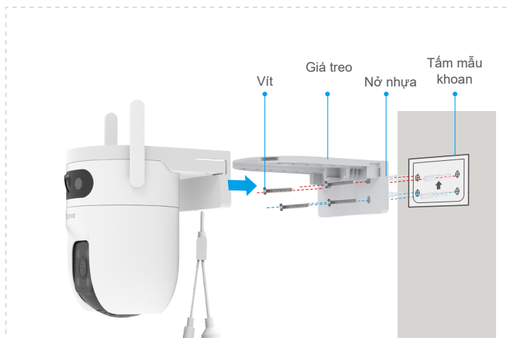
Hình 2 Gắn tường
